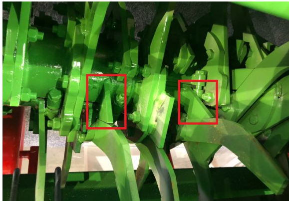
Extra svetsad stödtriangel för knivarna.
